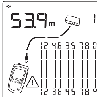
c) Kablo 3 ve 4 karışmış
