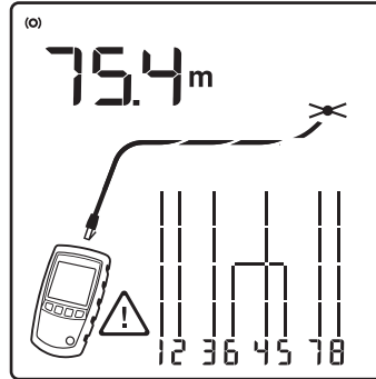
b) Kablo 6 ve 5 kısa devre
