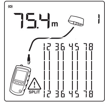
e) Ayrık çiftler
