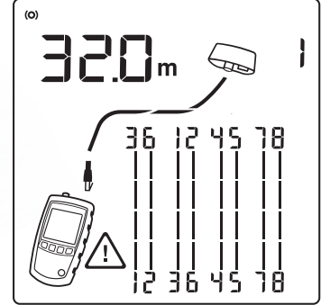
d) 1-2 ve 3-6 telleri karışmış
