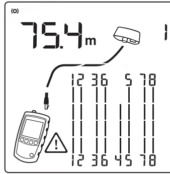
a) Kablo 4 blendajında açık devre
